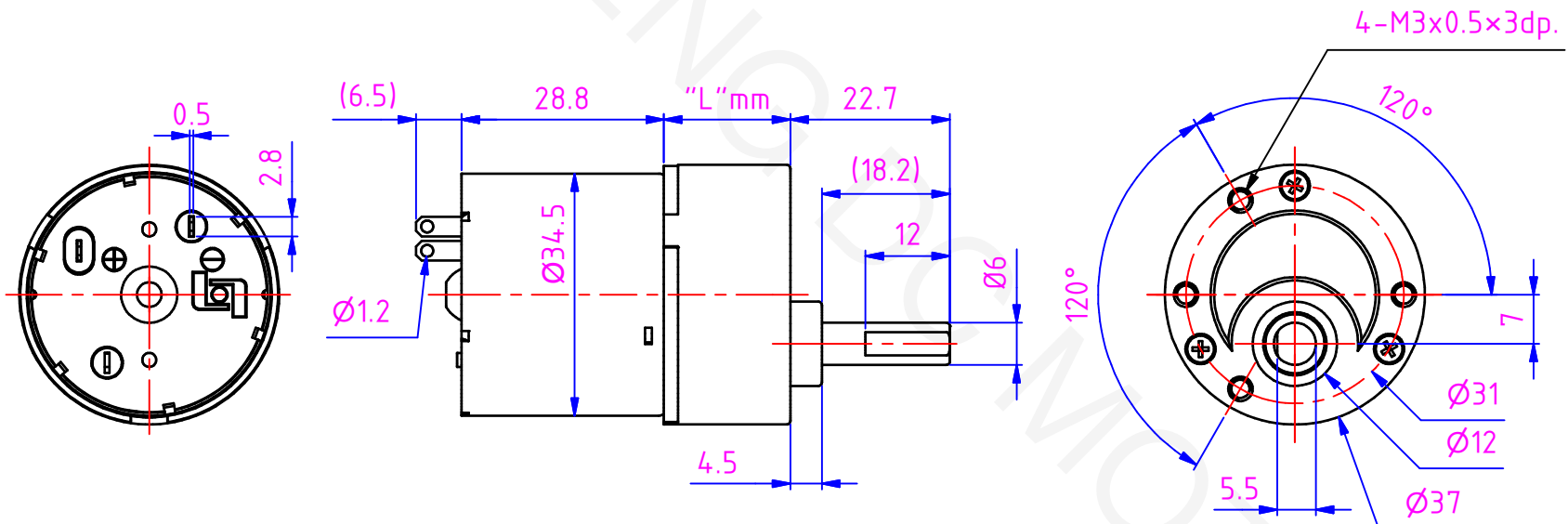
※HN35GMA TYPE
